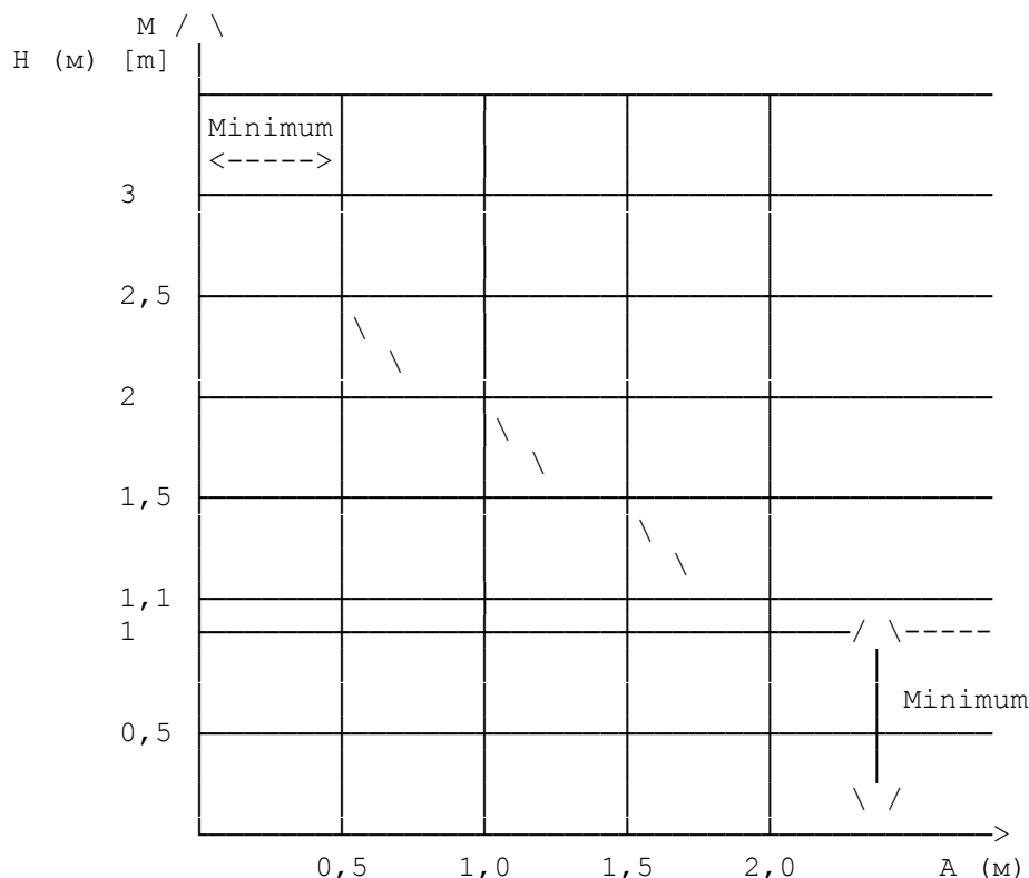
Рис. 1. Расстояние до движущихся элементов лифта
